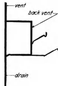
back vent
