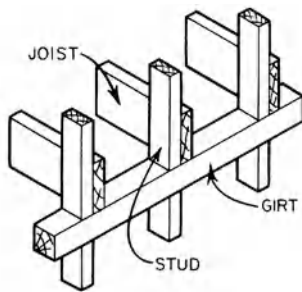
girt, 2
