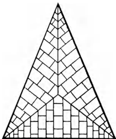
tripartite vault
