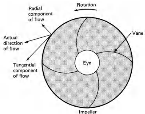
impeller
