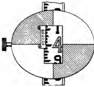
rod target
