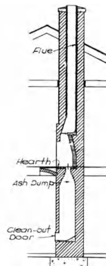
chimney
