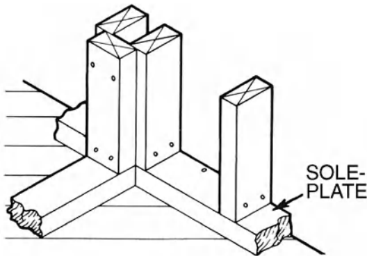
soleplate, 2
