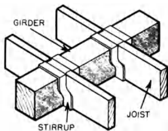
stirrup, 4
