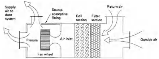
plenum fan
