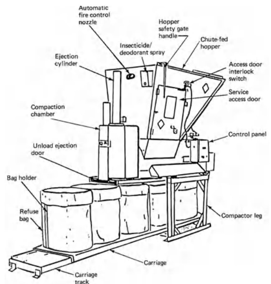
linear packer
