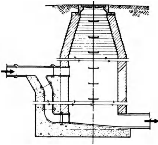
manhole
