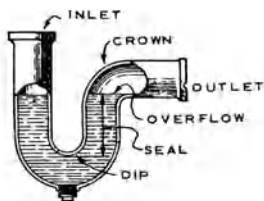
P-trap
