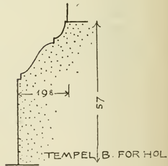
Fig. 8. Verschiedene Fussgesimsprofile von Podien.
